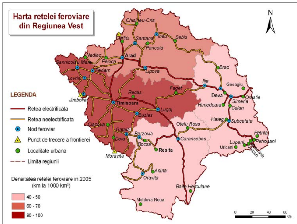
Figura III.1. Căile de transport feroviar și densitatea rețelei feroviare
