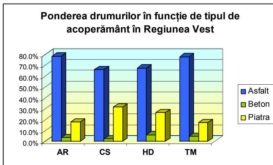
Figura III.2. Pondere drumurilor în funcție de tipul de acoperământ în Regiunea Vest Sursa: SC GAUSS SRL
